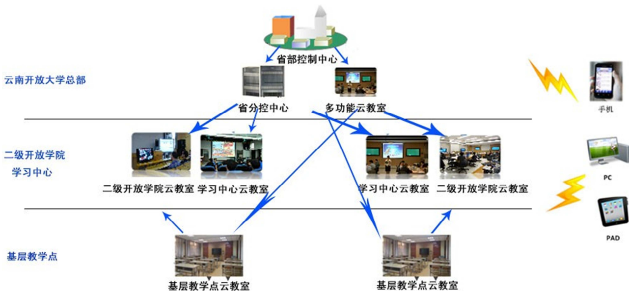
图1 云南开放大学云教室建设系统架构图。
